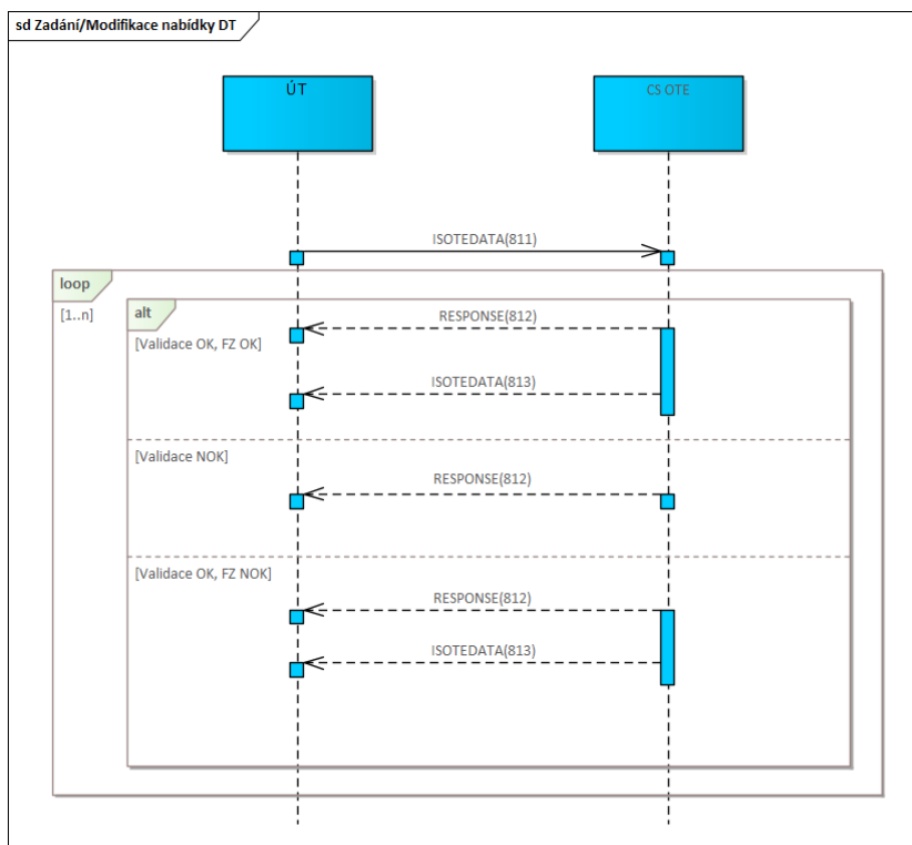
Obrázek 1 - Komunikační scénář - Zadáni/Modifikace nabídek na DT
